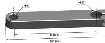
旋臂
