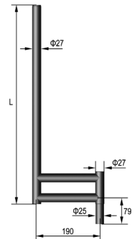
双臂钢管
