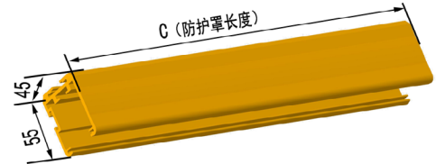
小型化光栅防护罩
