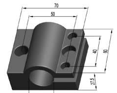
支架座
