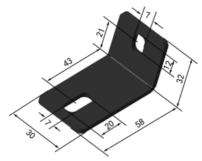
L 型弯板支架
