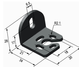
正侧装支架
