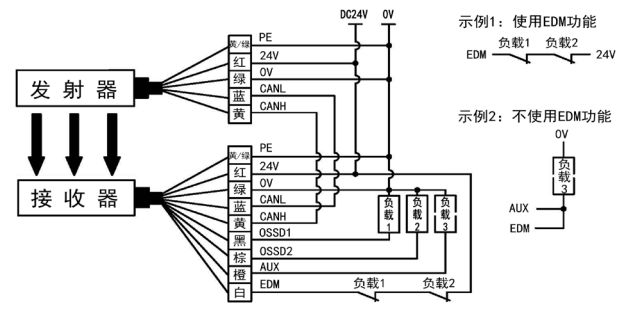
(3) PNP，线同步
