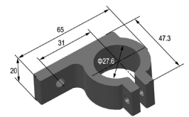
Q 型管夹
