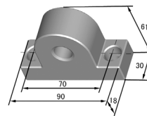
旋臂座
