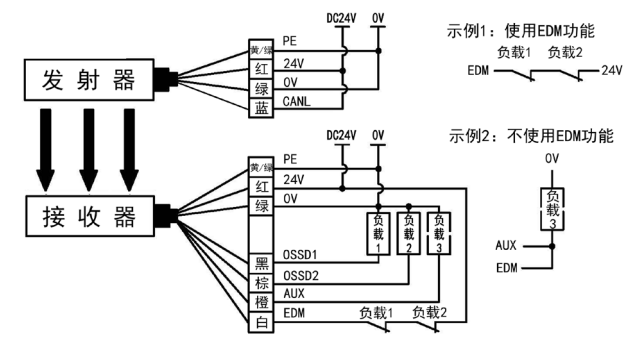
(3) PNP，线同步
